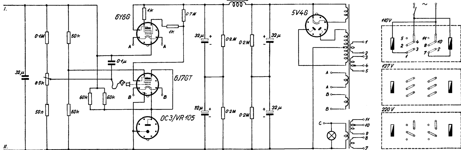
554. 54. ábra. Az EMG 1151 típusú impulzusgenerátor kapcsolási rajza
